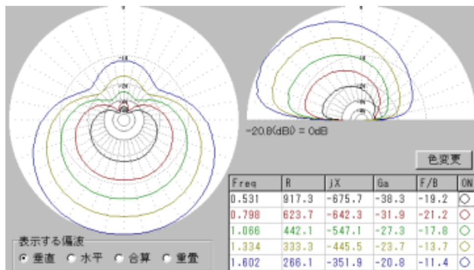
9. H=3m, L=20m, R_t=1520\ \Omega
